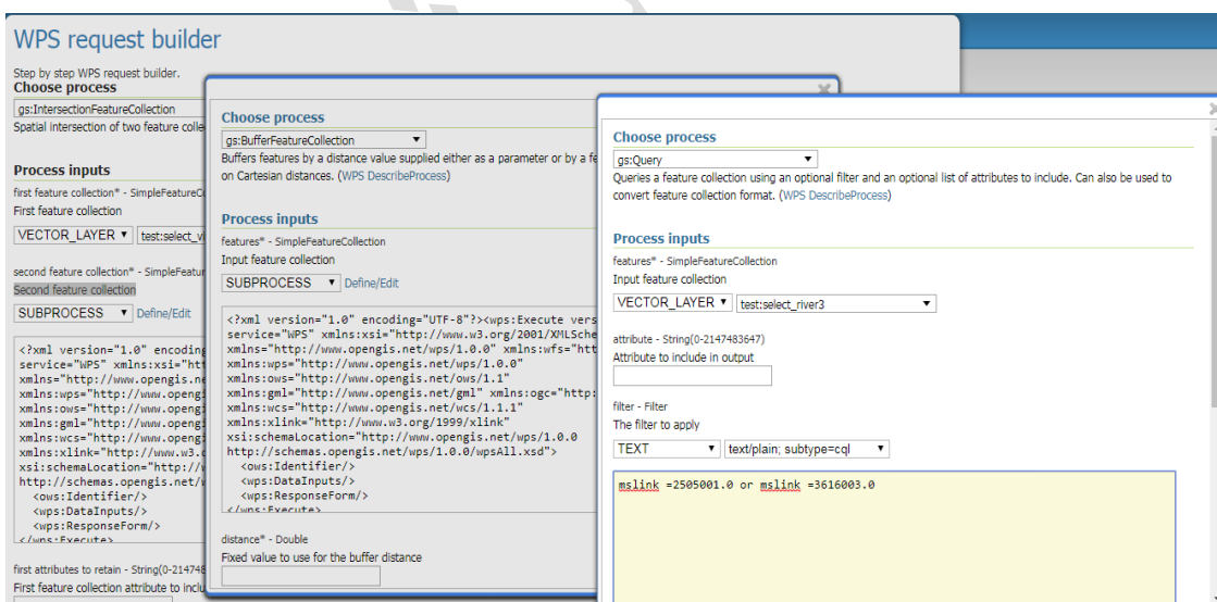
شکل ۷۲- وارد کردن کوئری مورد نظر به منظور انتخاب رودخانه جابجود
