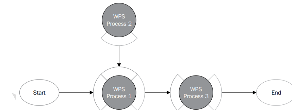
شکل ۱۴- Process Chaining
