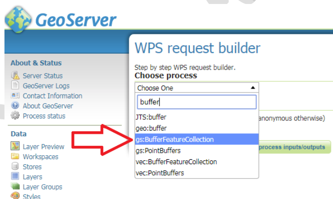
شکل ۲۵- انتخاب تحلیل Buffer از منوی Choose process
