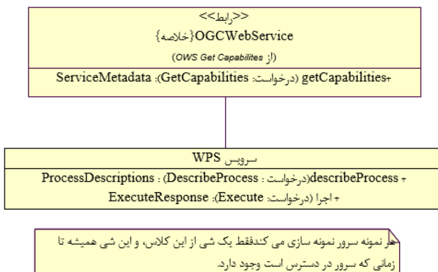
شکل ۱۳- نمودار UML رابط WPS
