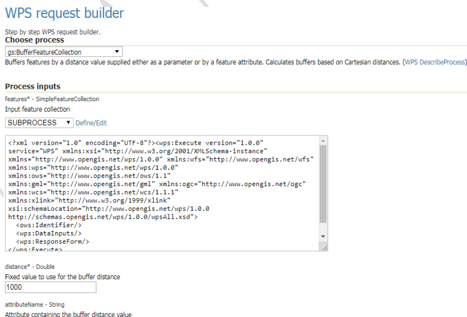
شکل ۶۹- فایل XML حاصل از تحلیل Query به عنوان ورودی تحلیل Buffer
