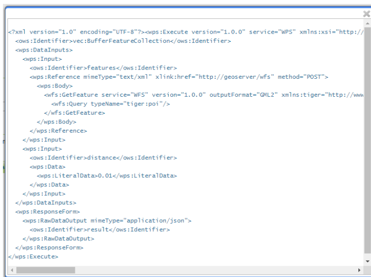
شکل ۳۲- دریافت خروجی تحلیل Buffer در زبان XML
