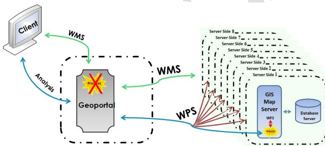
شکل ۷۶- ساختار پیشنهادی
