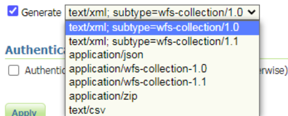
شکل ۳۳- نمایش انواع فرمت خروجی تحلیل های WPS در نرم افزار GeoServer
