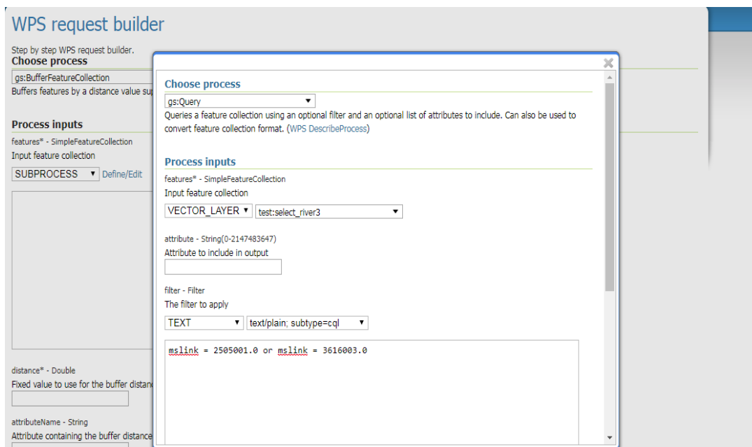
شکل ۶۸- انتخاب تحلیل Query به عنوان ورودی تحلیل Buffer
