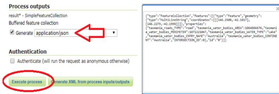
شکل ۴۱- انتخاب فرمت استاندارد مورد نظر به عنوان خروجی تحلیل Intersection
